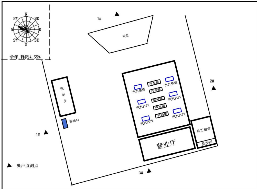
图 3-2 噪声监测点位示意图
