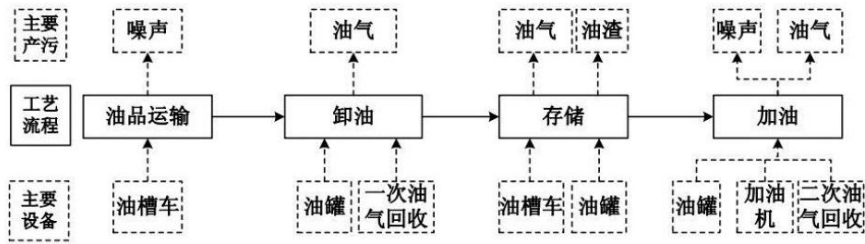
图 1-1 生产工艺流程图
