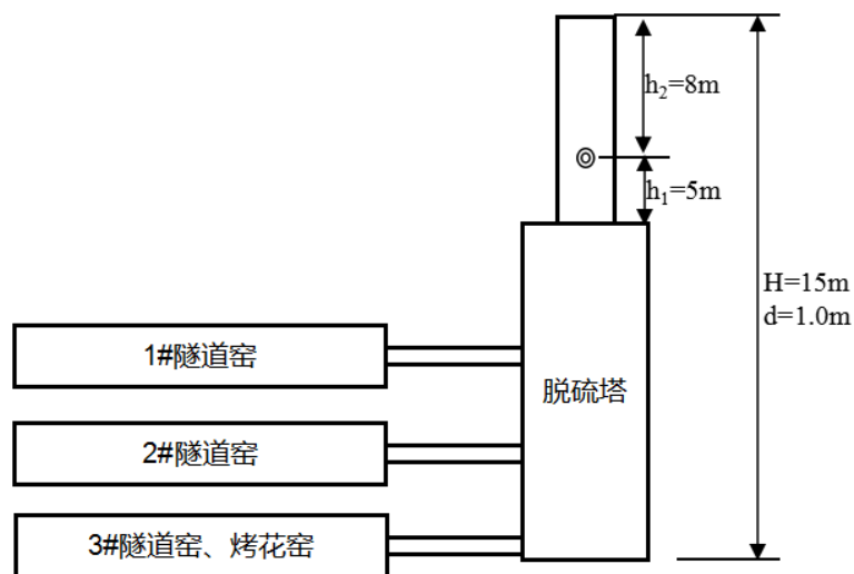
图 3-4 窑炉废气总排放口监测点位示意图
