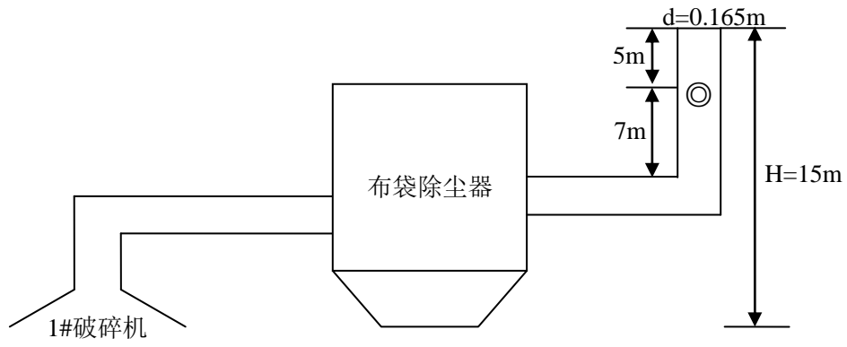
图3-1 1#破碎机废气排放口监测点位示意图
