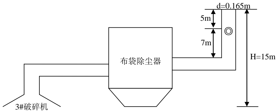
图 3-2 2#破碎机废气排放口监测点位示意图
