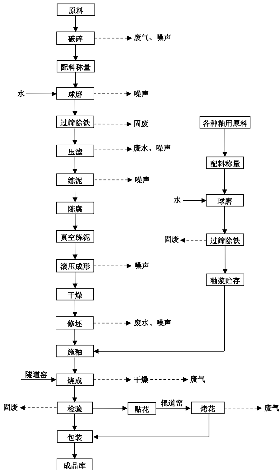
图1-1 本项目工艺流程图
