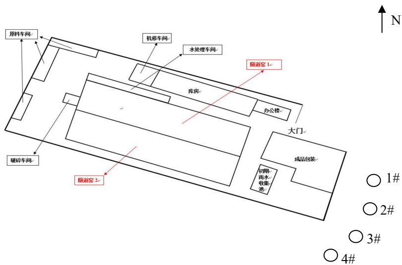
图3-2 隧道窑废气总排放口监测点位示意图
