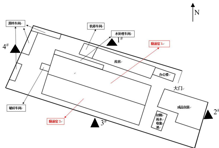
图 3-5 厂界噪声监测点位示意图
