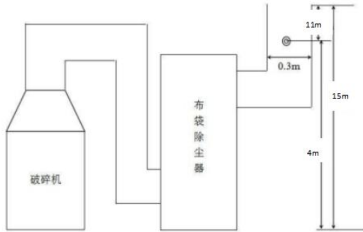
图 3-2 破碎除尘器监测点位示意图 (DA002)
