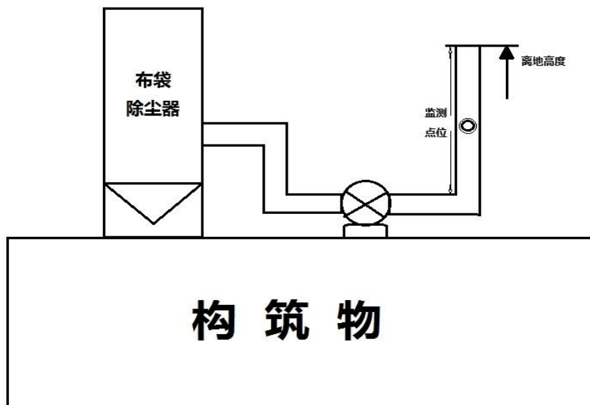
图 3-4 一般排放口的有组织颗粒物监测点位示意图
