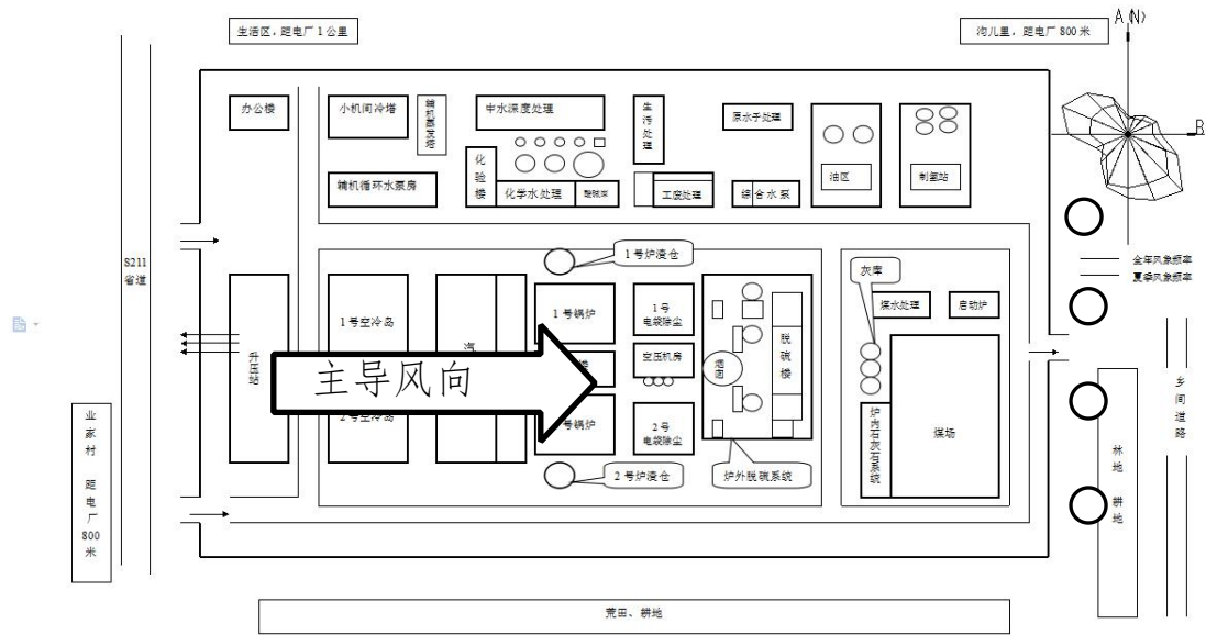
山西京玉发电有限责任公司厂区示意图
