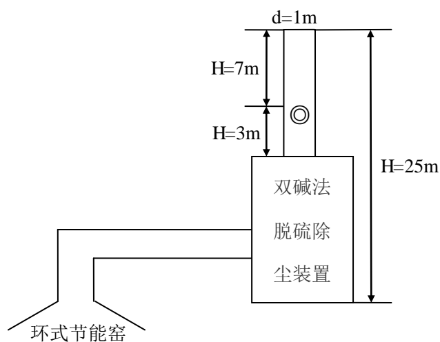
图 3-1 环式节能窑废气排放口监测点位示意图
