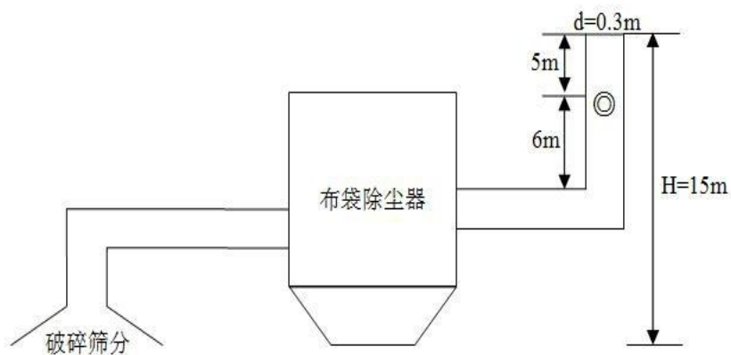
图3-2 破碎筛分废气排放口监测点位示意图
