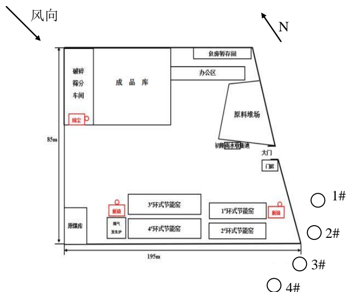
图 3-3 厂界无组织监测点位示意图
