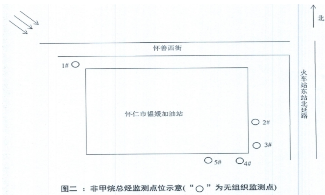
图 3-2 无组织废气监测点位示意图
