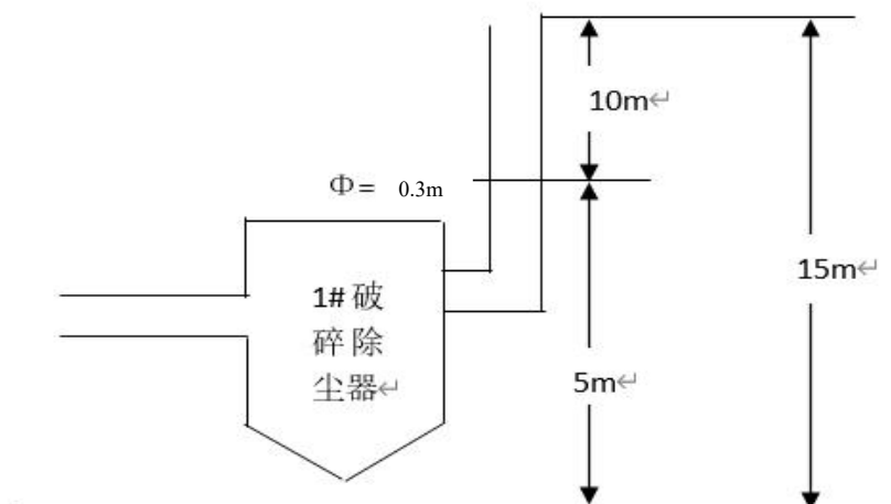
图 1 1#破碎废气手工监测点位示意图
