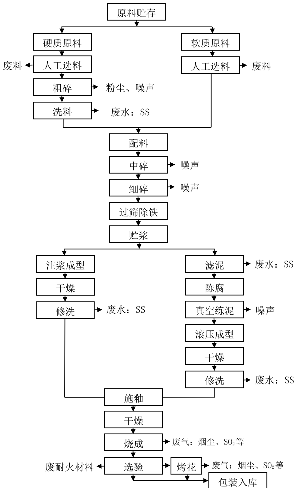
图 1 排污环节流程图
