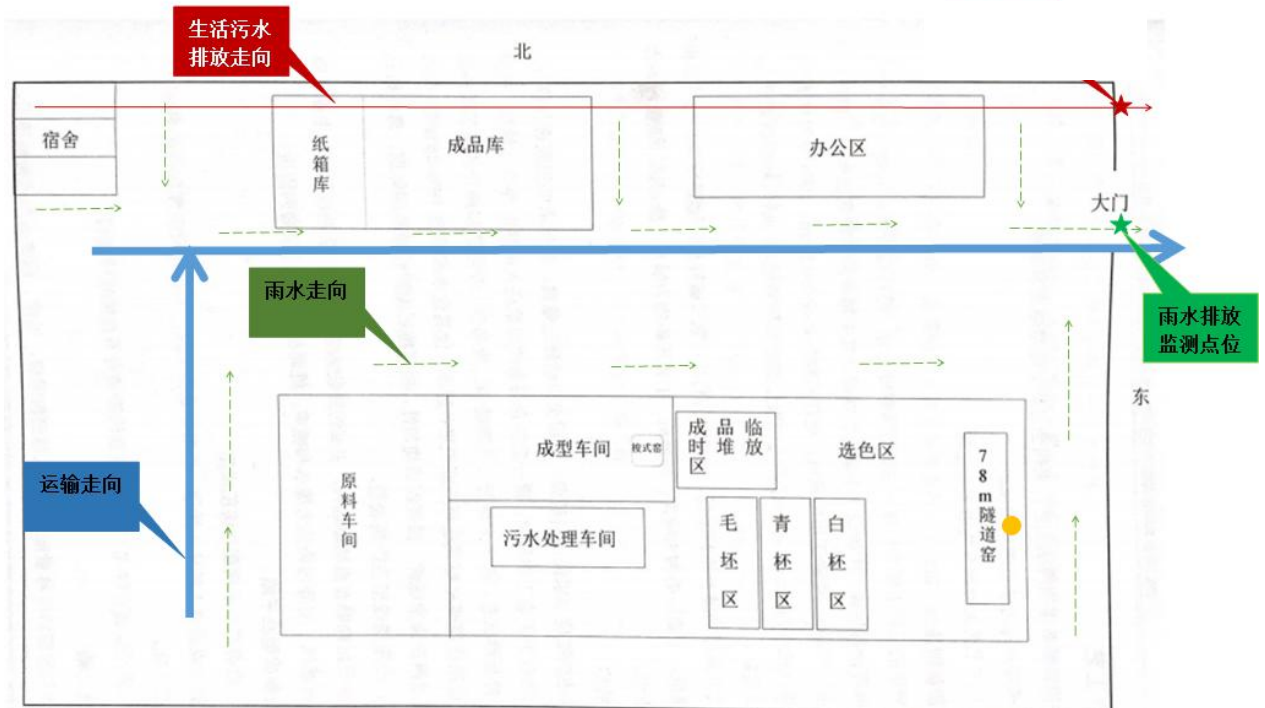
图 3-4 废水监测点位示意图
