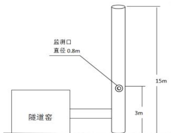
图 3-2 隧道窑烟气监测点位图
