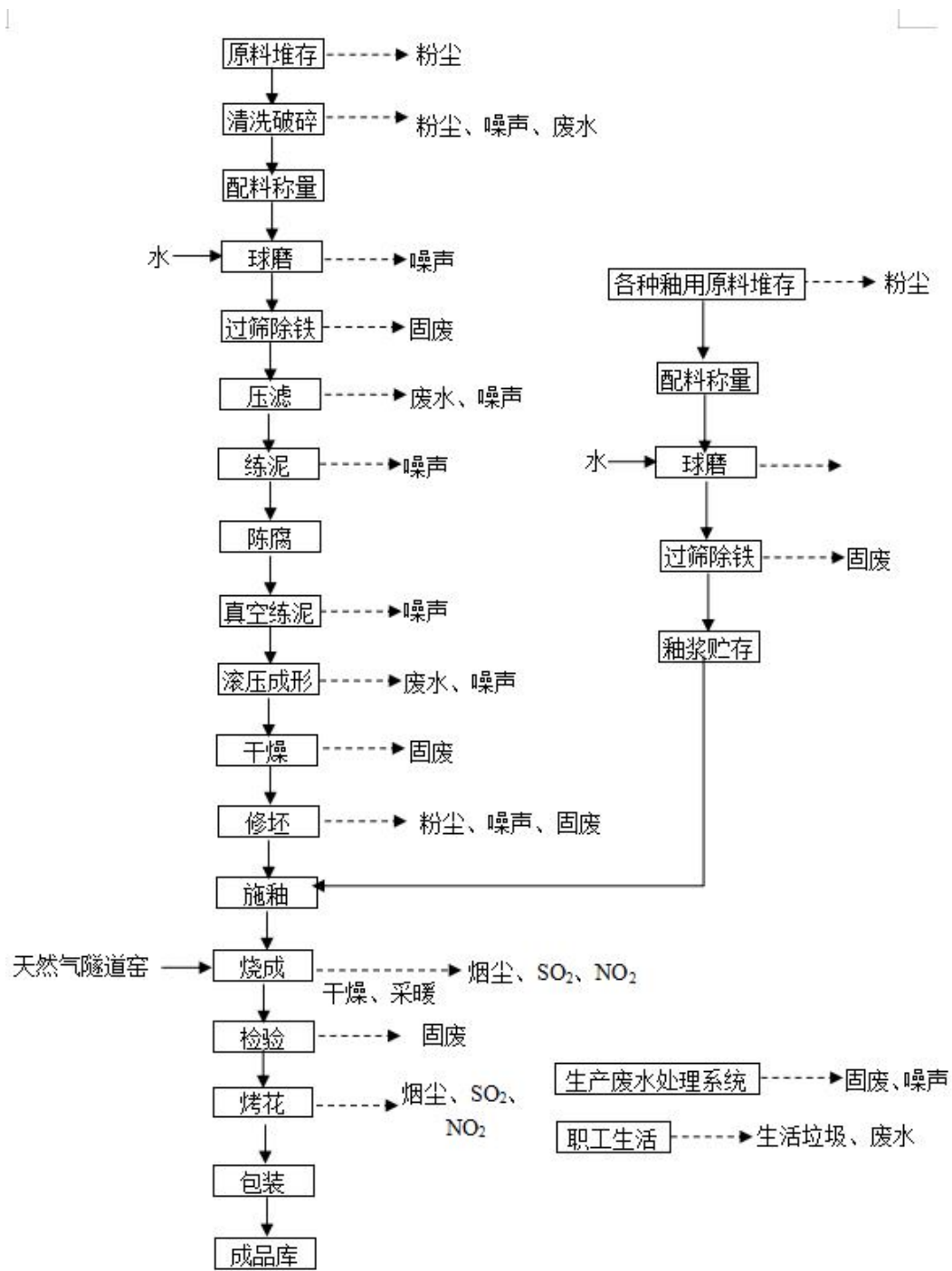
图 1-1 生产工艺流程图及产污节点
