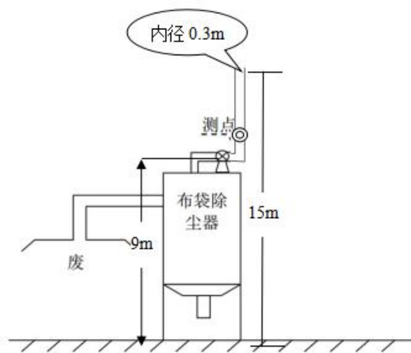
图 3-1 布袋除尘器监测点位图
