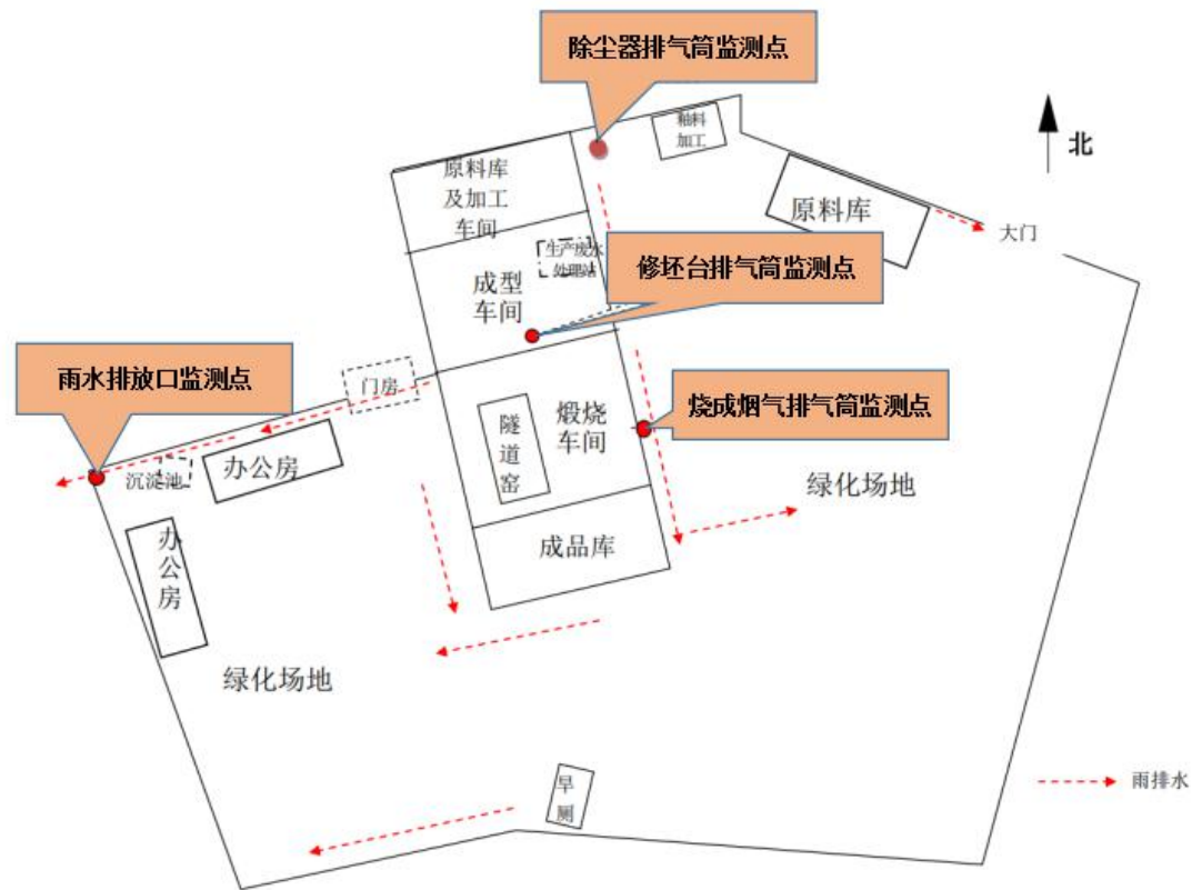
图 3-4 废水监测点位示意图
