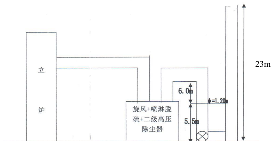
图 3-2 立窑废气监测点位示意图 (DA001~DA006)
