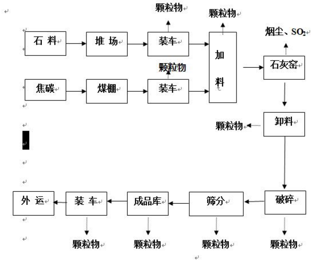
图 1-1 生产工艺及产污节点流程图
