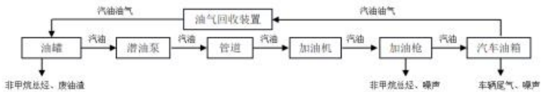
图 1-2 汽油加油与产污工艺流程图
