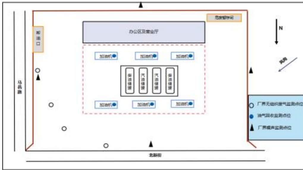
图 3-1 中国石化销售股份有限公司山西朔州神朔路加油站监测点位布设图 (注: 以实际监测时气象条件为准)
