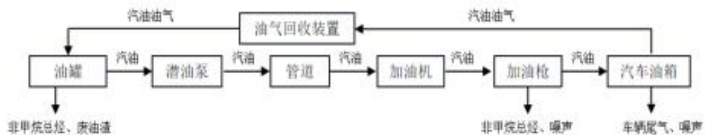
图 1-2 汽油加油与产污工艺流程图
