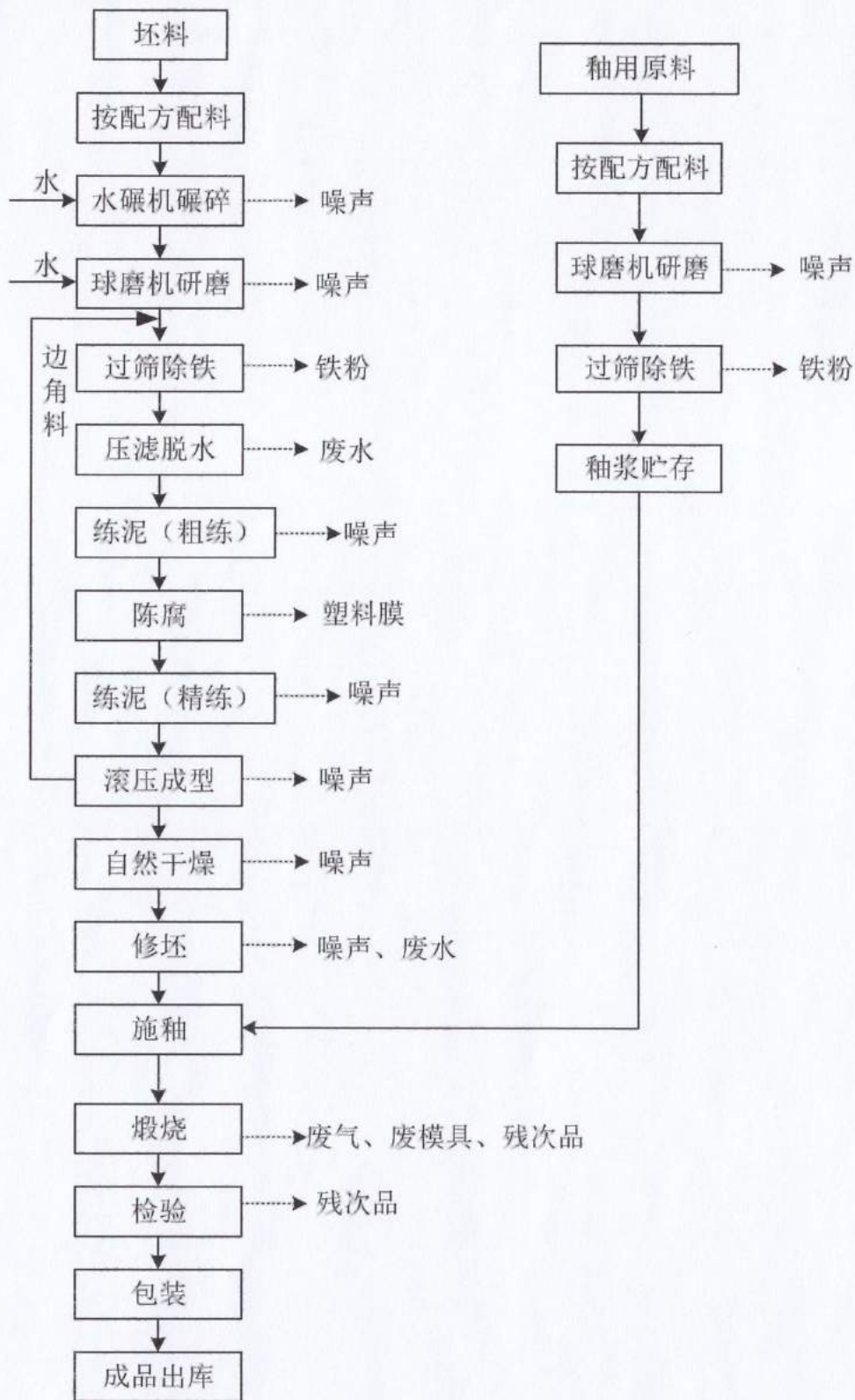
图 1.2-1 工艺流程图
