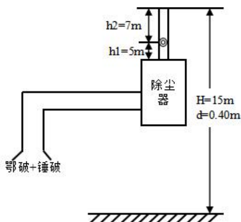
图3-2 破碎废气排放口监测点位示意图
