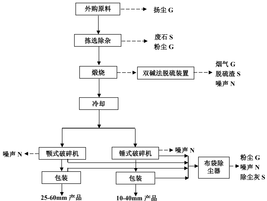
图1-1 本项目工艺流程图
