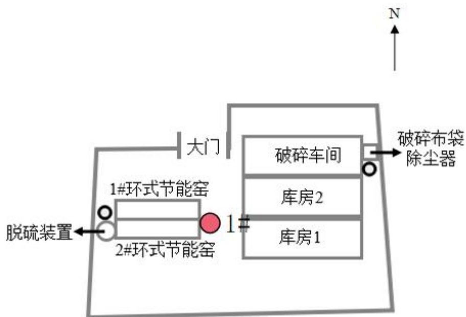
图 3-3 工业炉窑周边无组织监测点位示意图
