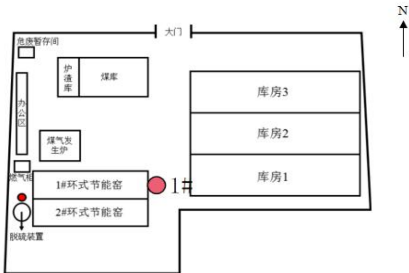
图 3-2 工业炉窑周边无组织监测点位示意图
