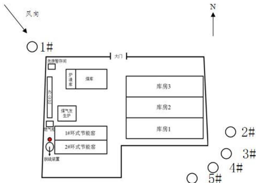
图 3-3 厂界无组织监测点位示意图
