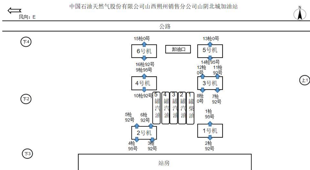
图2 无组织监测点位示意图
