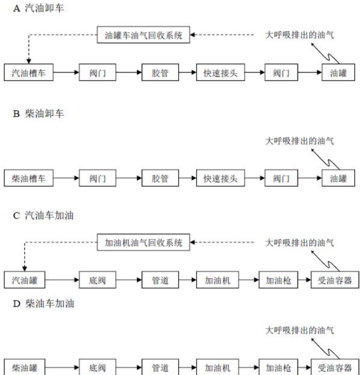
图1 工艺流程图
