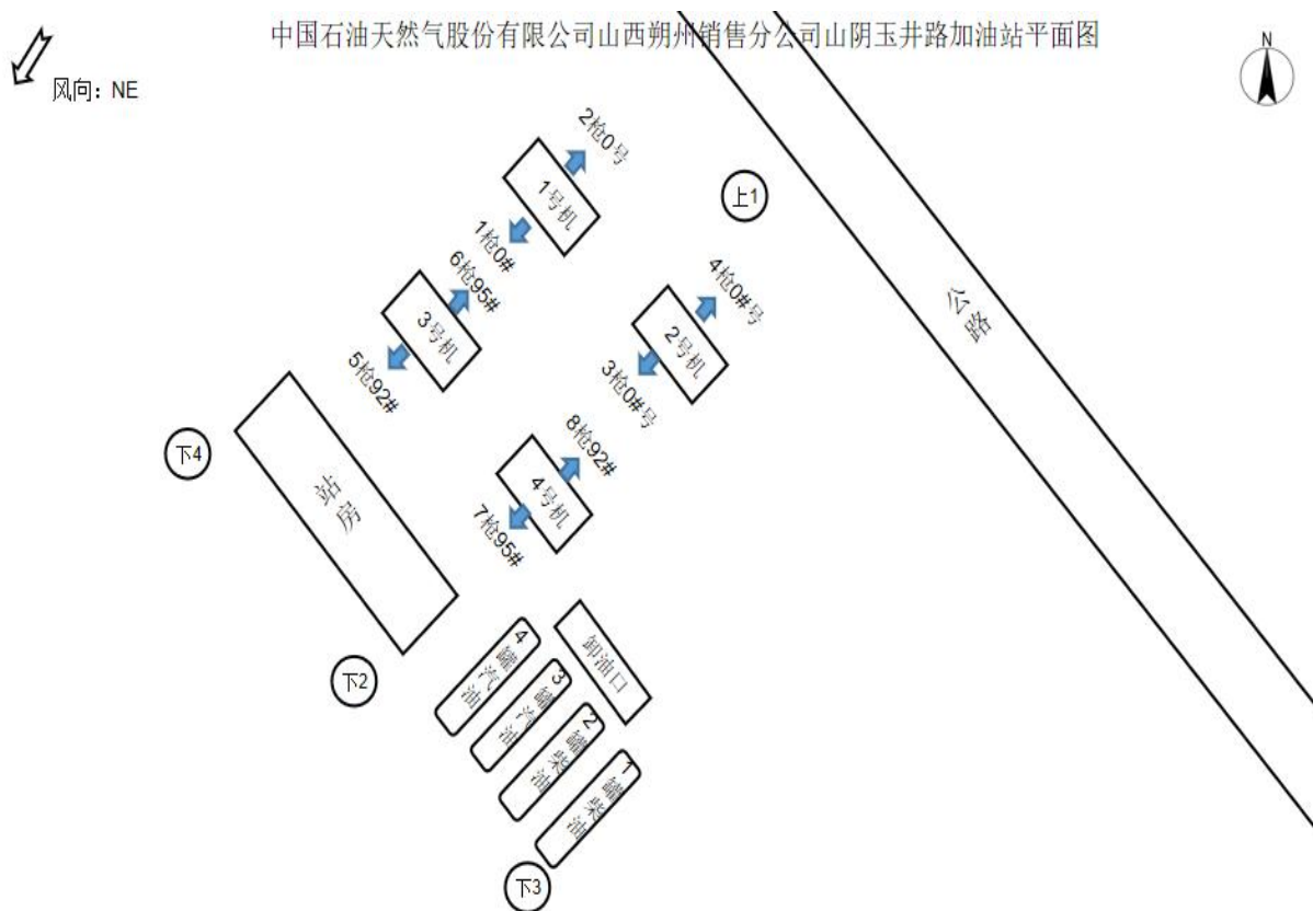
图2 无组织监测点位示意图
