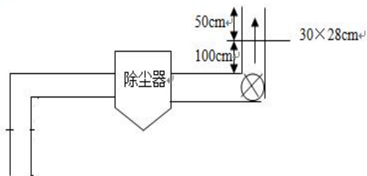
图 3-3 配料库库顶除尘器监测点位示意图
