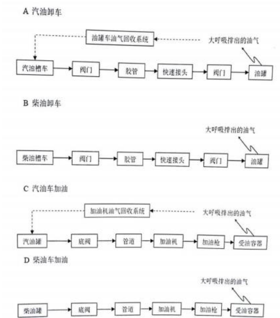
图 1 工艺流程图
