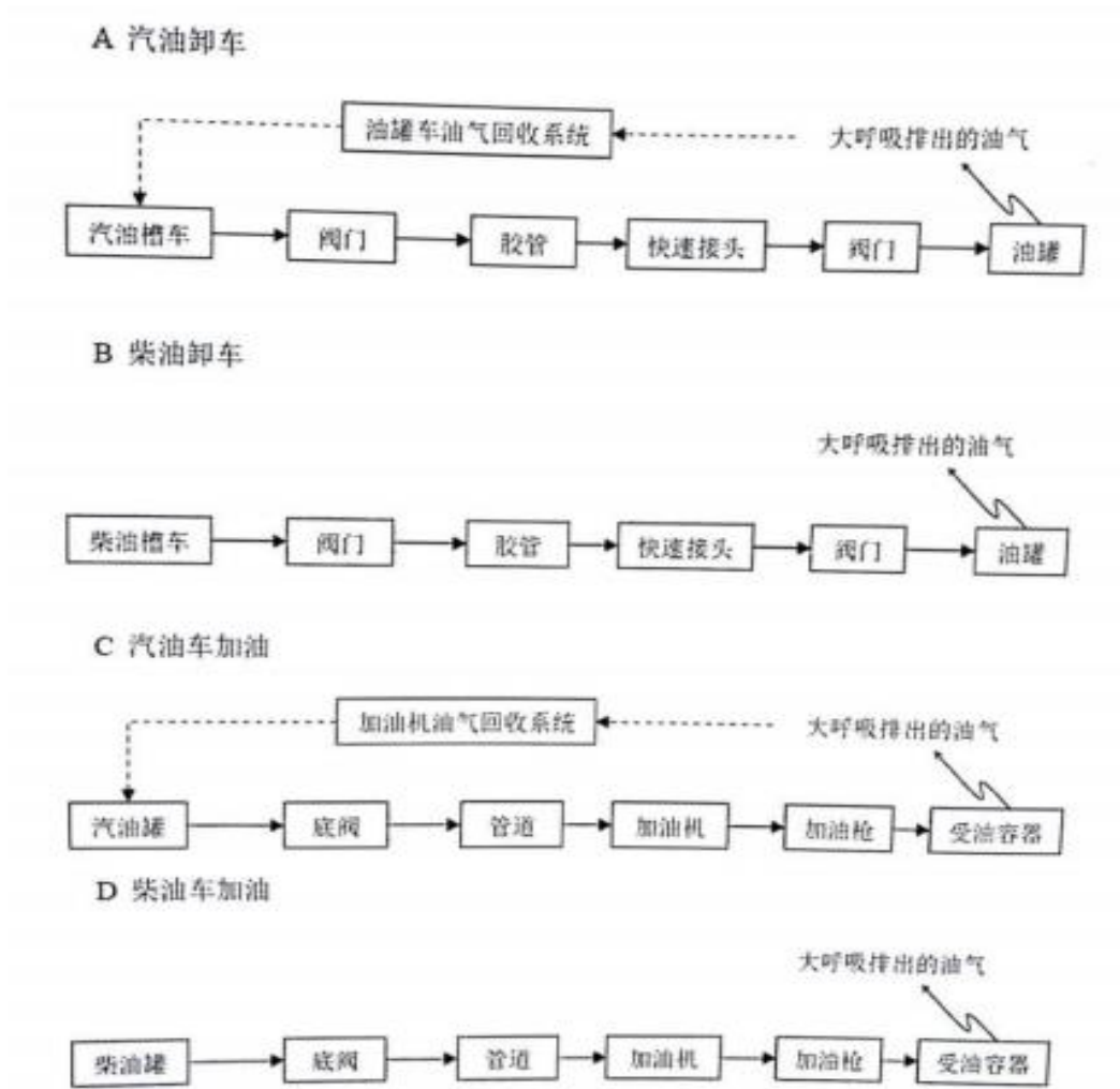
图 1 工艺流程图
