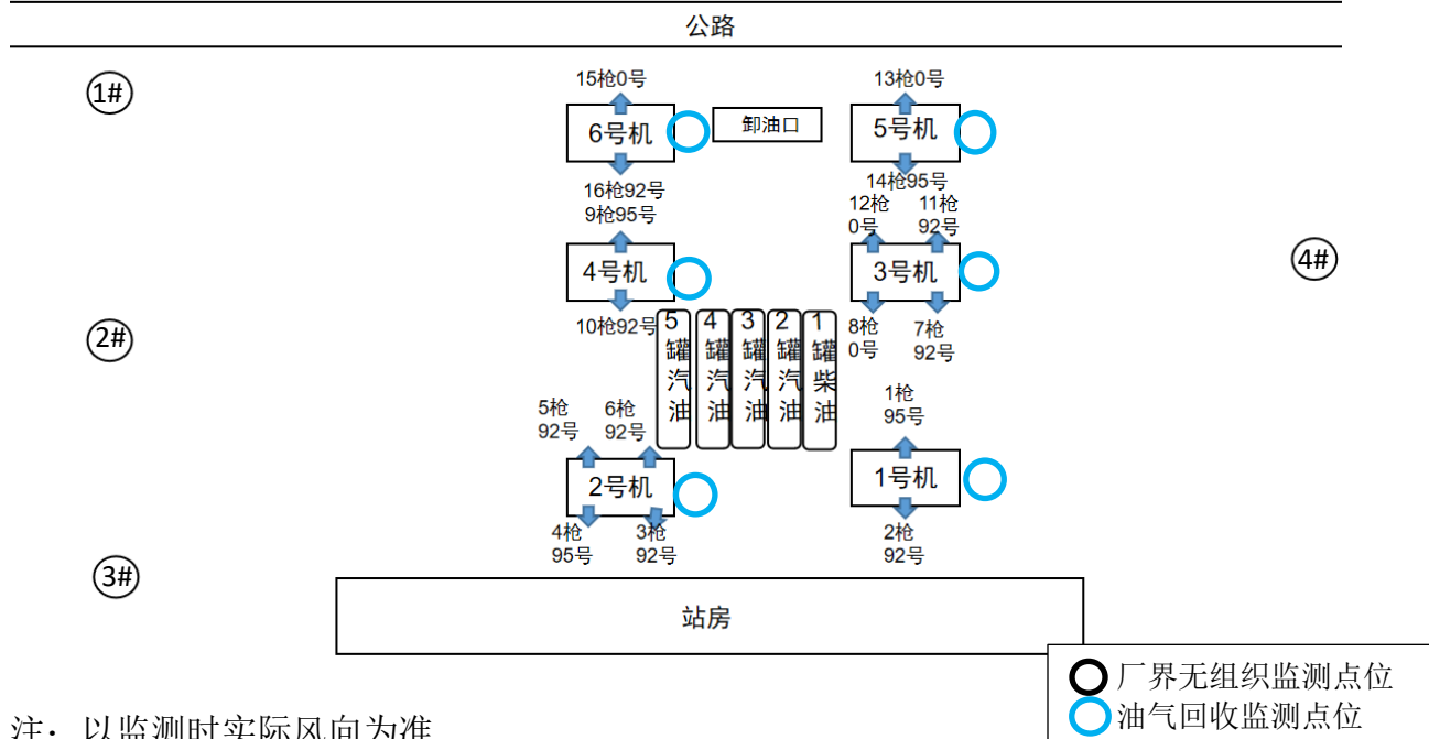
图 2 监测点位示意图
