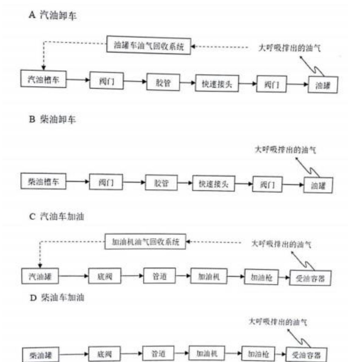
图 1 工艺流程图
