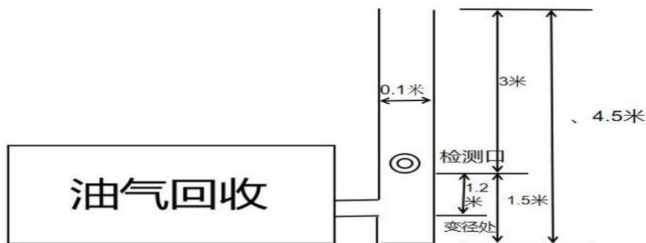
图 3 有组织废气监测点位示意图
