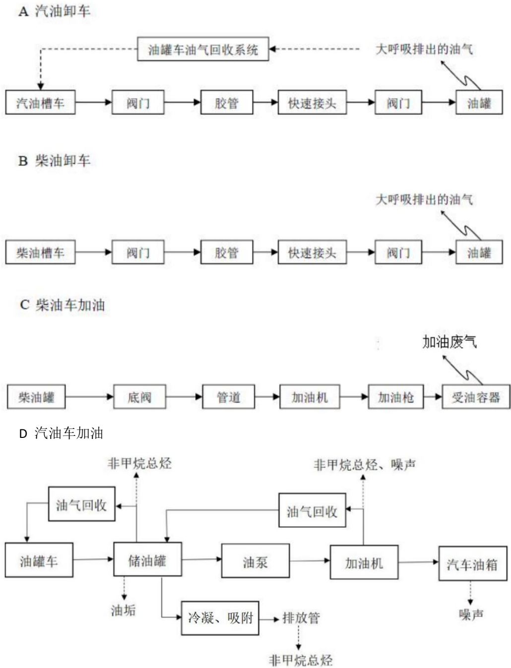
图 1 工艺流程图
