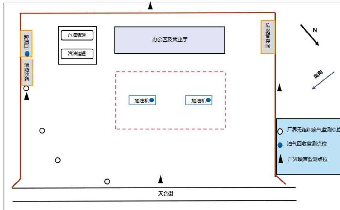
图 3-1 中国石化销售股份有限公司山西朔州怀仁怀应路加油站监测点位布设图
