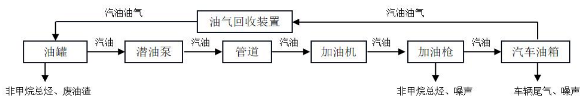
图 1-2 汽油加油与产污工艺流程图
