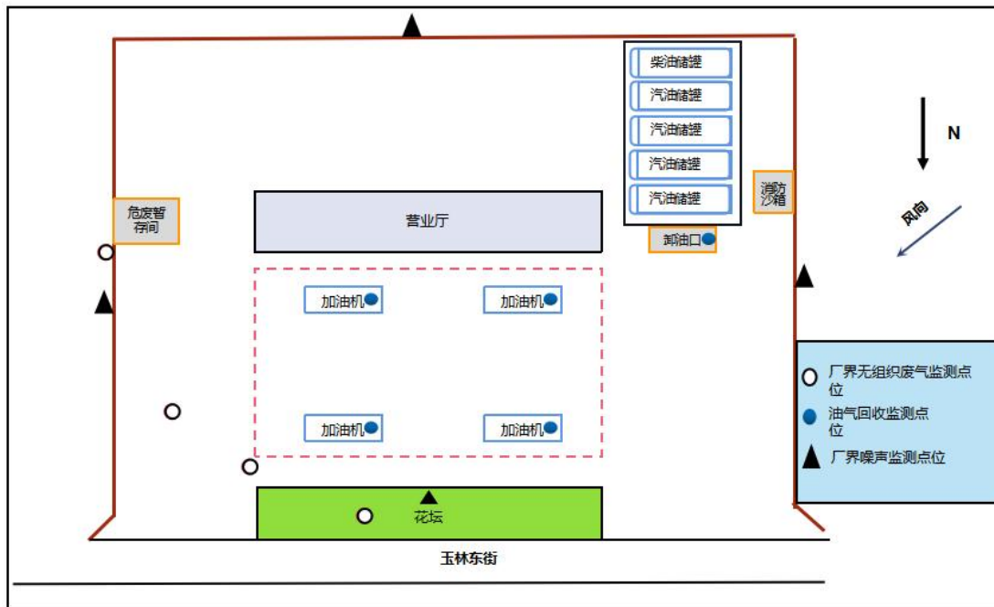
图 3-1 中国石油化工股份有限公司山西朔州右玉上堡加油站监测点位布设图
