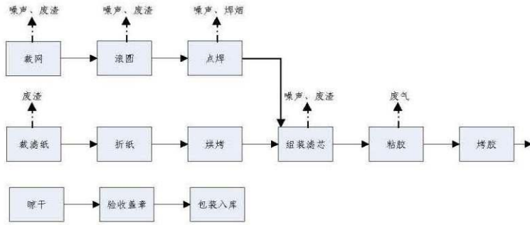
图 2-5 滤清器生产工艺流程
