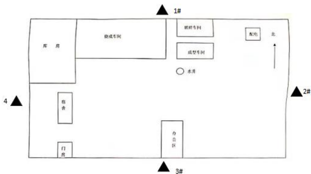
图 3-4 工业场地噪声监测布点示意图
