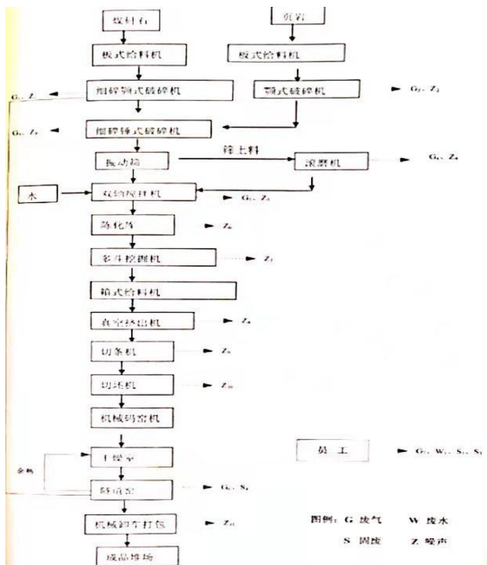
图 1-1 工艺流程图
