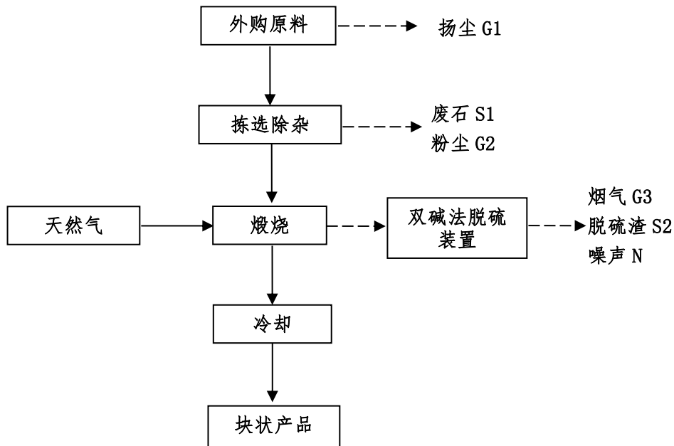
图 1-1 本项目工艺流程图
