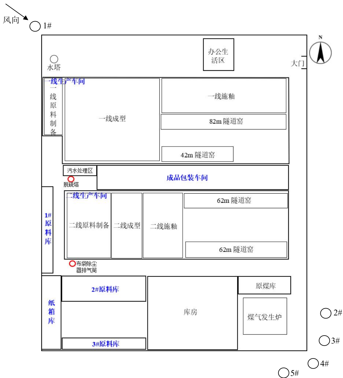
图3-3 厂界无组织监测点位示意图
