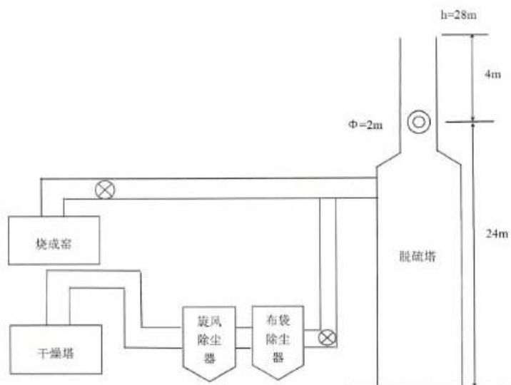
图3-4 2#喷雾干燥塔、烧成窑废气总排放口监测点位示意图
