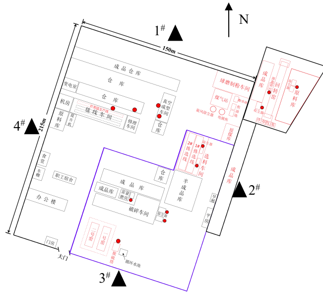
图 3-8 厂界噪声监测点位示意图
