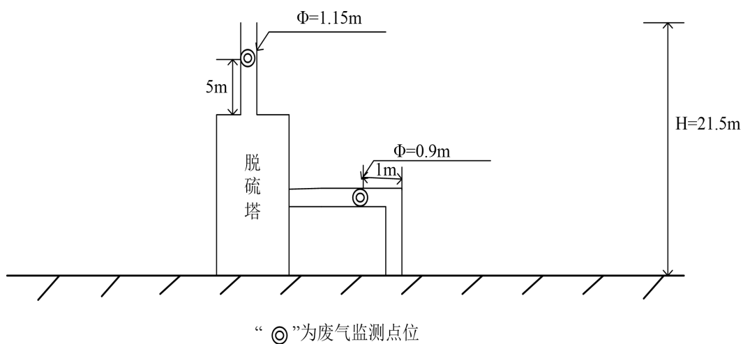
图 3-3 环式节能窑烟气排放口监测点位示意图
