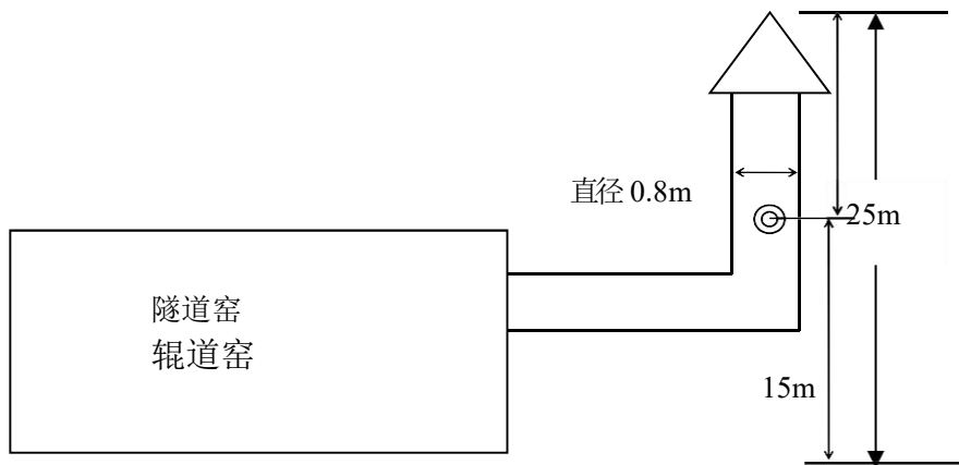
图 3-2 隧道窑废气监测布点示意图
