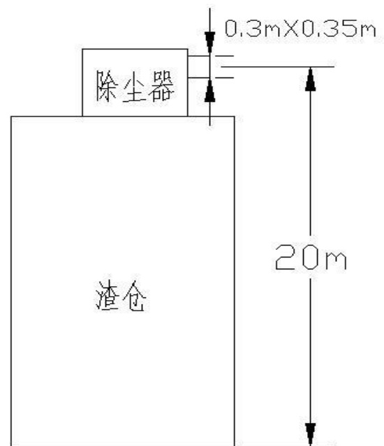
图3-11 渣库排口监测点位示意图
