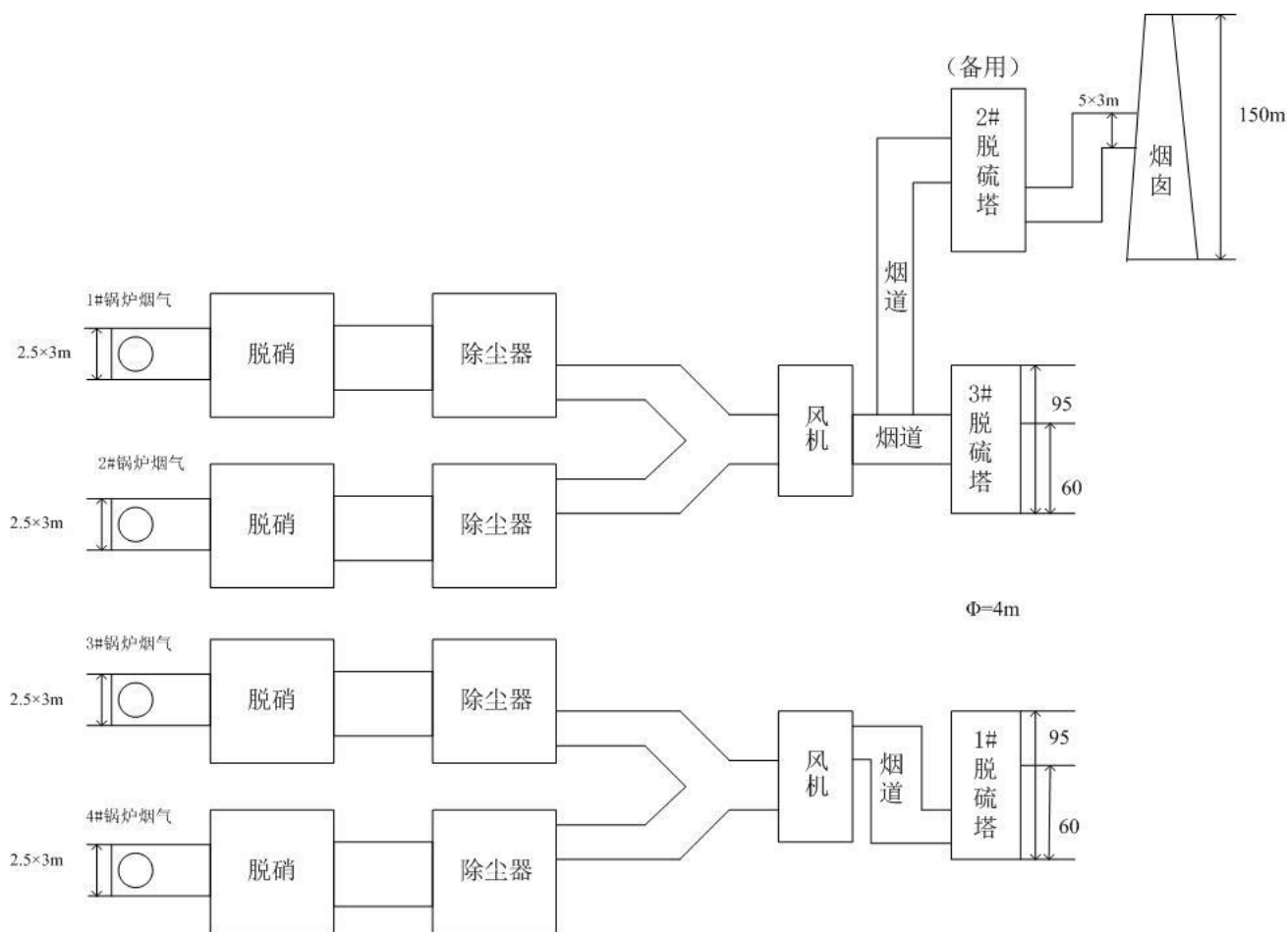
图3-1 动力锅炉脱硫塔出口监测点位示意图
