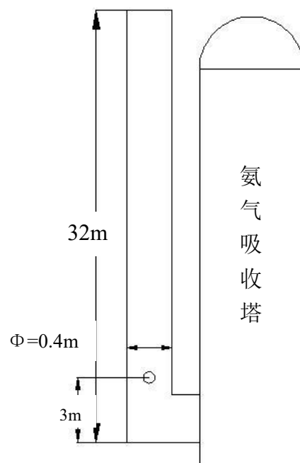
图3-13 氨气吸收塔排口监测点位示意图
