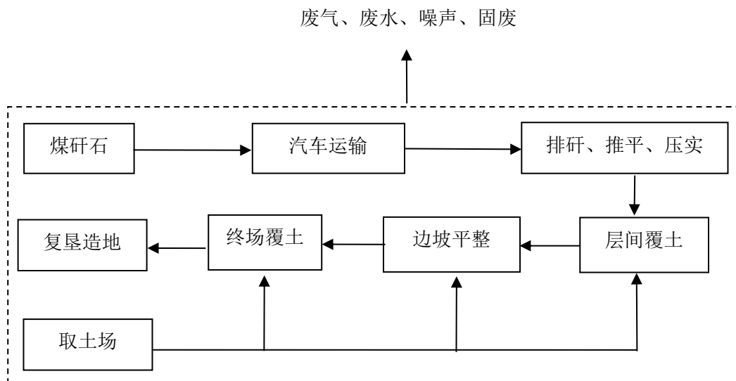
图 1-1 填沟造地工艺流程图及产排污环节
