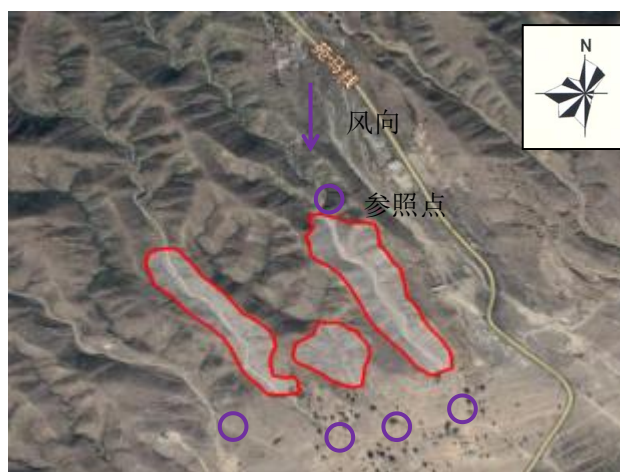
图 3-1 无组织废气监测点位图
