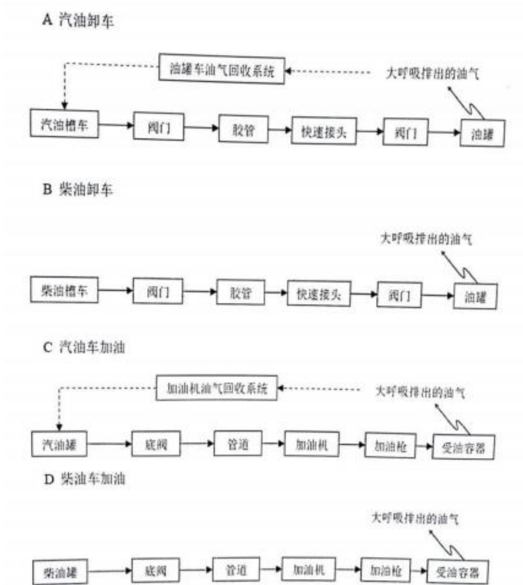
图 1 工艺流程图
