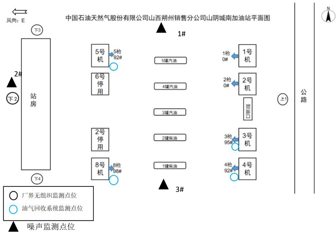
图 2 无组织废气监测点位示意图
