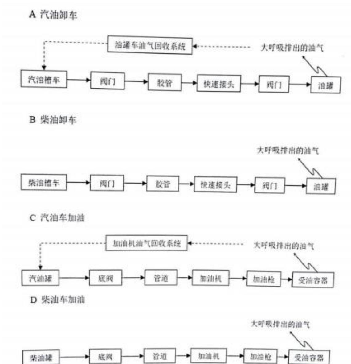
图 1 工艺流程图
