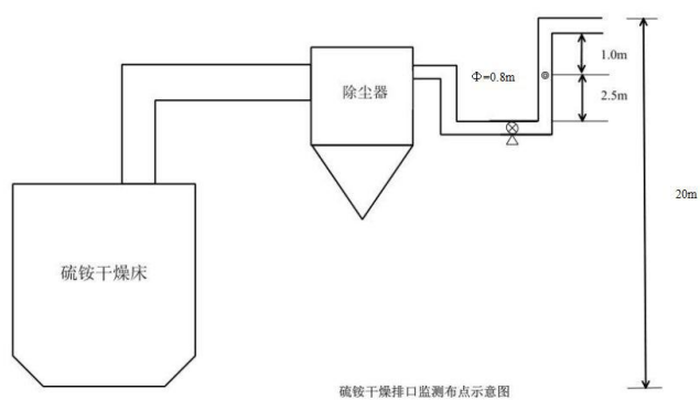
图3-4 硫铵干燥排口监测点位示意图
