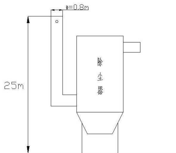
图3-3 硝铵包装机1#、2#排口监测点位示意图
