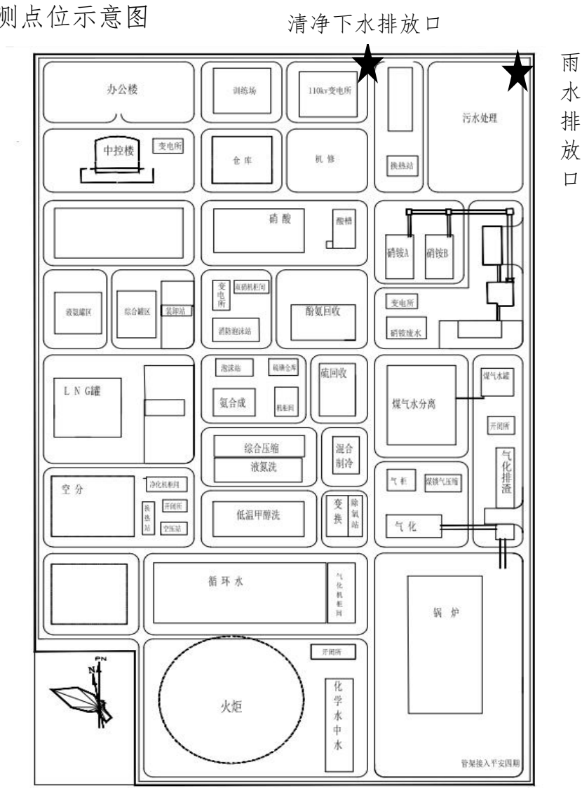
图 3-17 劣质煤项目生产区废水监测点位示意图
