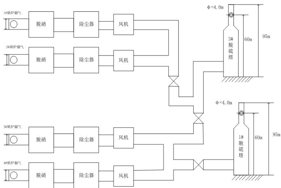
图3-1 动力锅炉脱硫塔出口监测点位示意图
