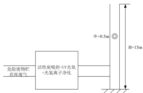
图3-15 危险废物贮存库废气排口监测点位示意图
