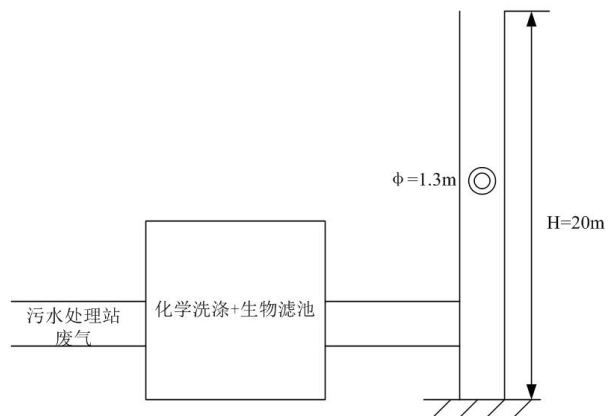
图3-14 污水处理站废气排口监测点位示意图
