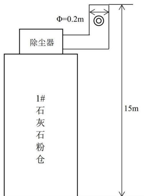
图3-11 石灰石仓排口监测点位示意图
