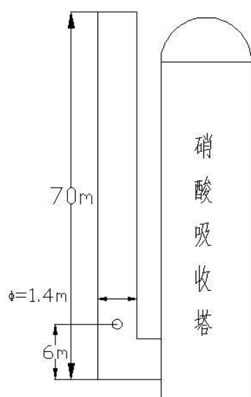
图3-8 1#、2#硝酸尾气排口监测点位示意图
