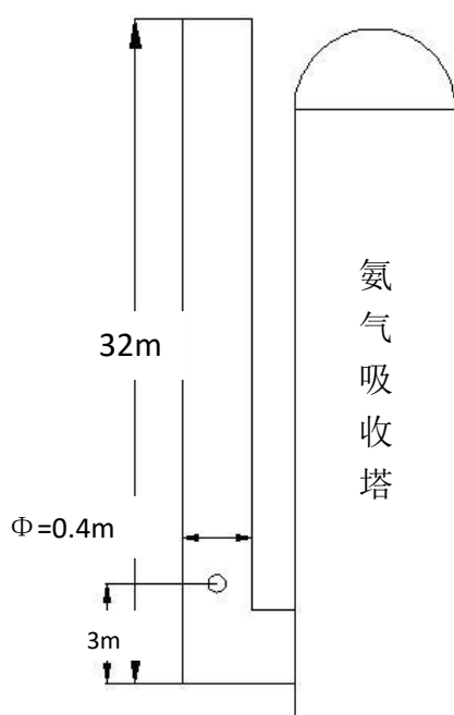
图3-12 氨气吸收塔排口监测点位示意图
