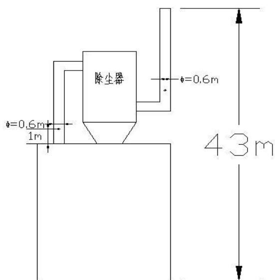
图3-2 原料气制备备煤筛分机排口监测点位示意图
