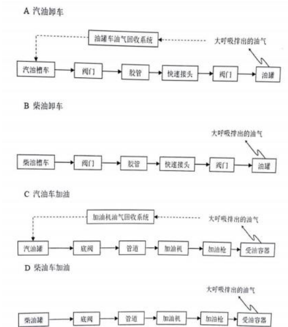
图 1 工艺流程图
