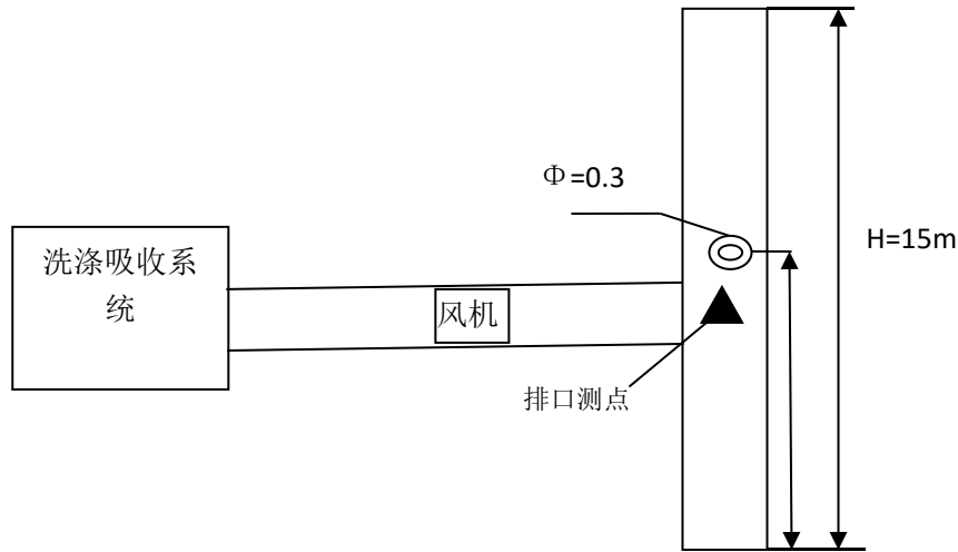
图 3-3 偏二甲肼废气排口监测点位示意图
