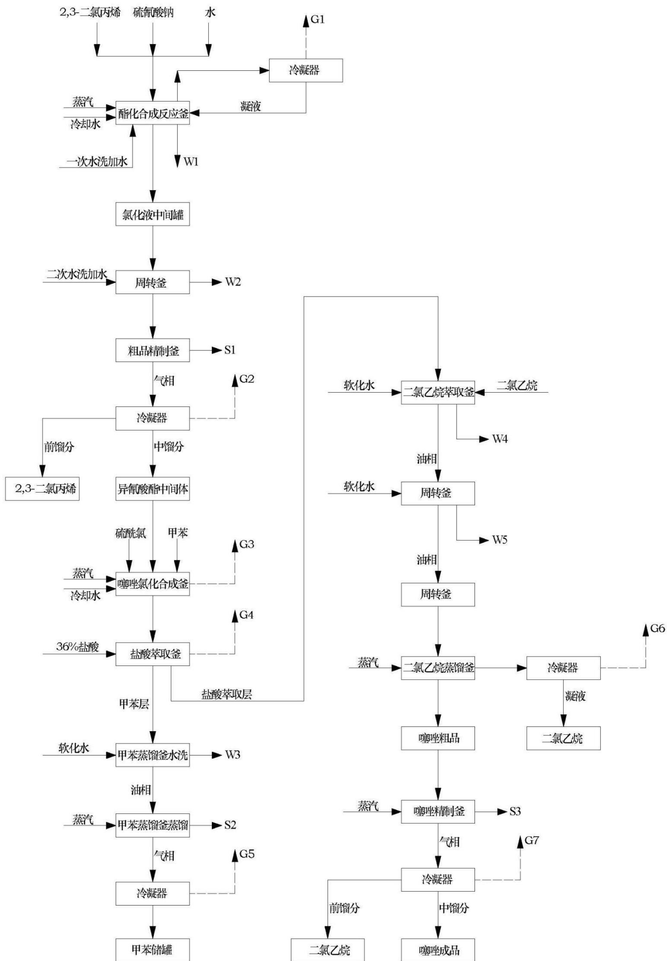
图 3 2-氯-5-氯甲基噻唑生产工艺流程图
