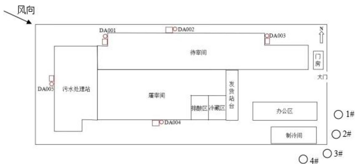
图 3-6 厂界无组织废气监测点位示意图
