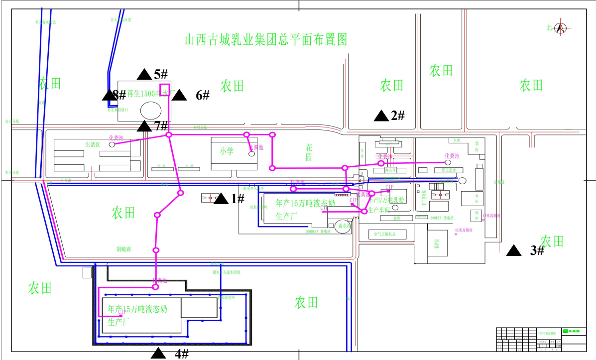
图 3-6 厂界噪声监测点位示意图
