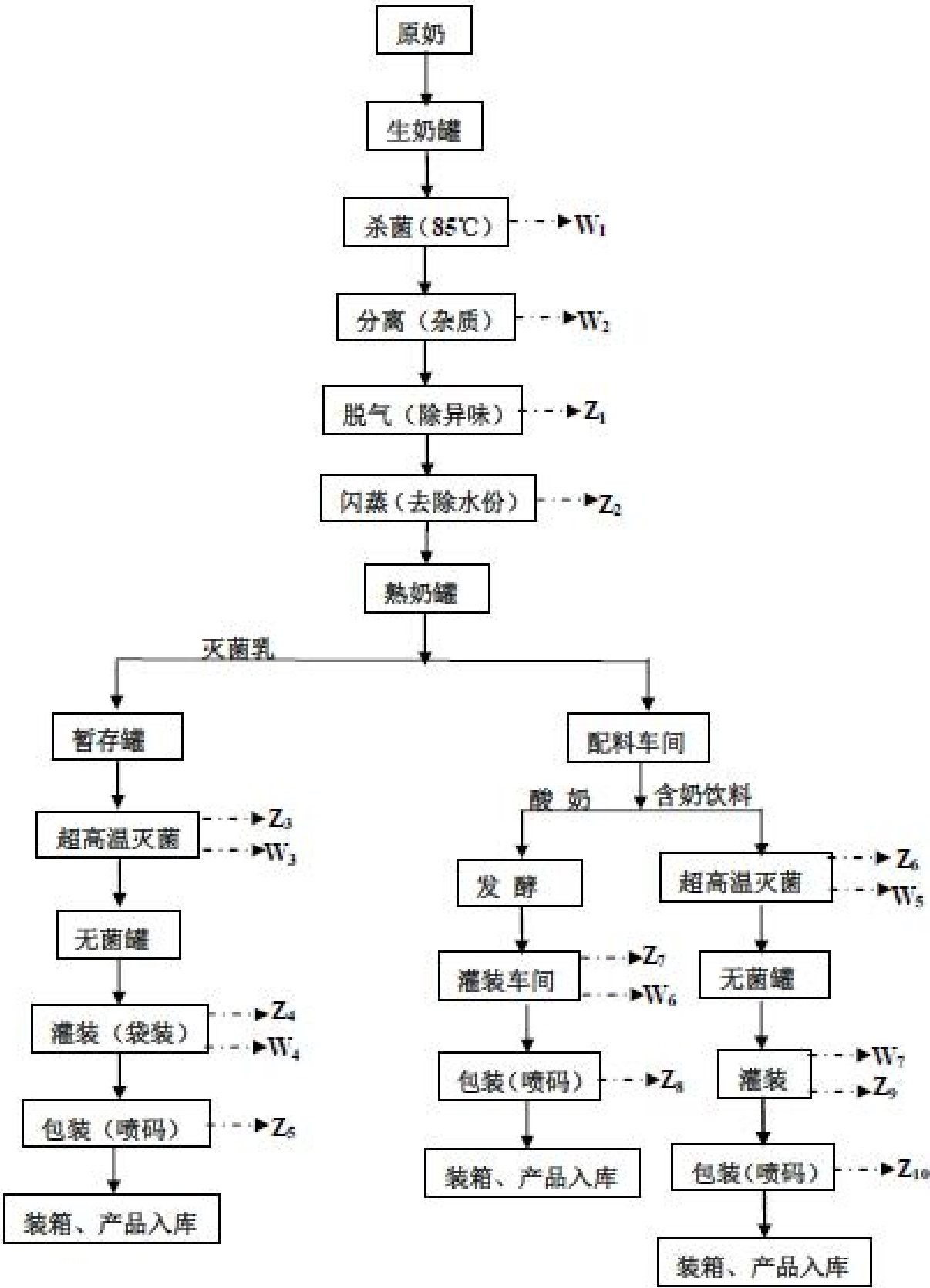
图1-3 年产15万吨液态奶生产工艺及产排污环节流程图
