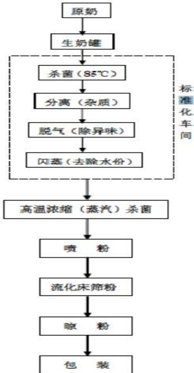
图1-1 年产1万吨固态奶粉生产工艺及产排污环节流程图
