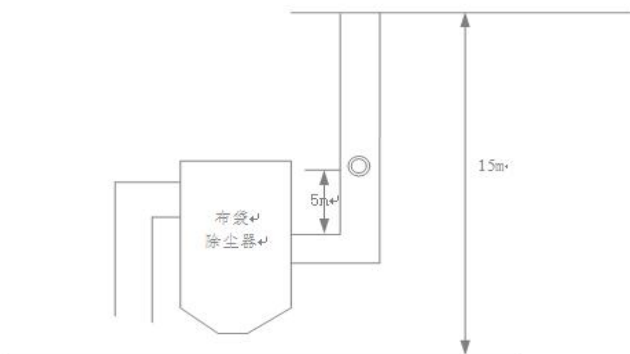
图 3-3 奶粉干燥废气排放口监测点位示意图 (DA001)
