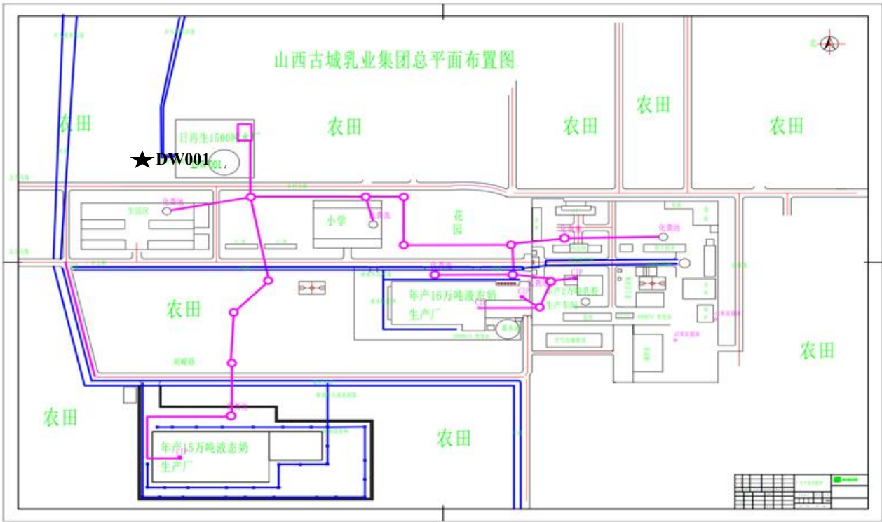
图 3-5 综合污水排放口监测点位示意图（DW001）
