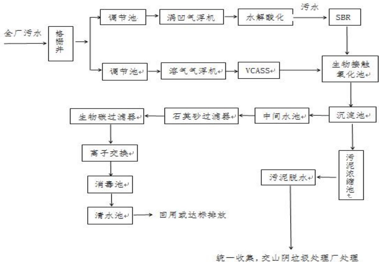
图1-4 综合污水处理站污水处理工艺流程图
