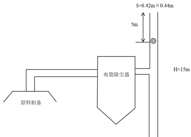
图3-3 3#原料干碾废气排放口监测点位示意图
