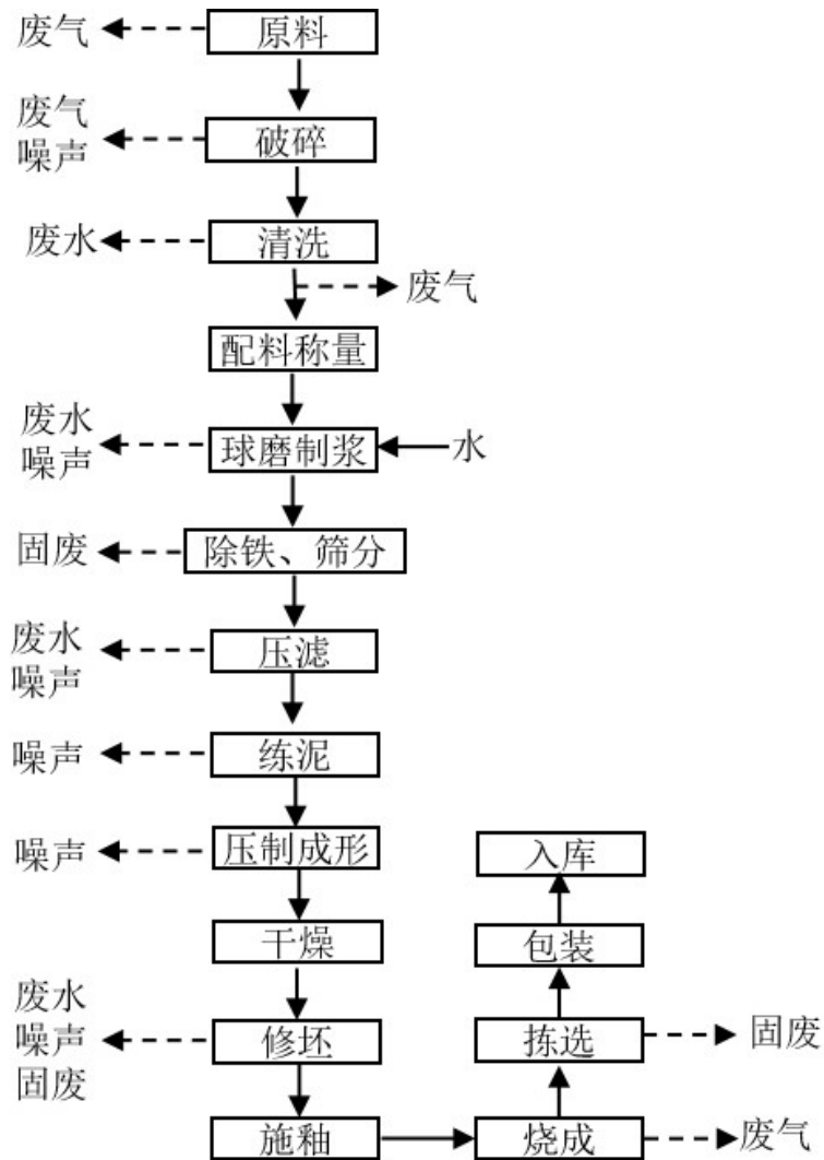
图1-1 本项目工艺流程图
