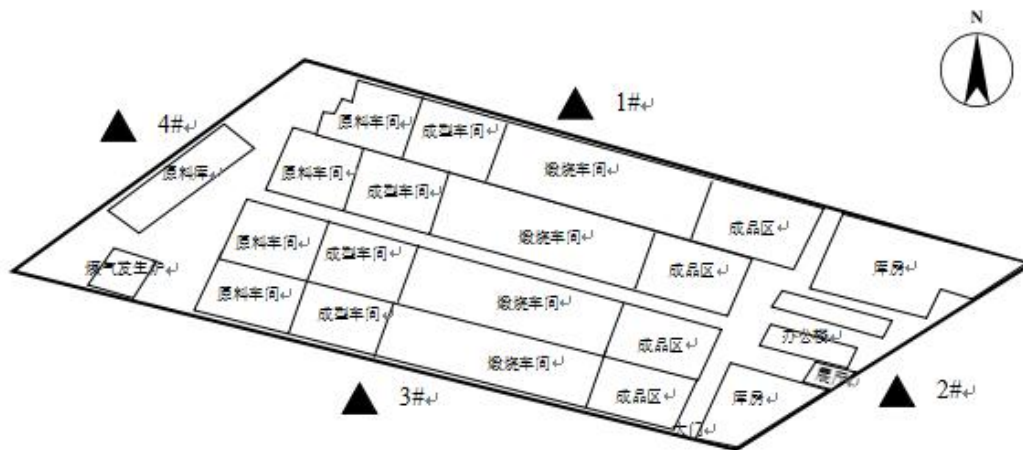
图 3-6 厂界噪声监测点位示意图
