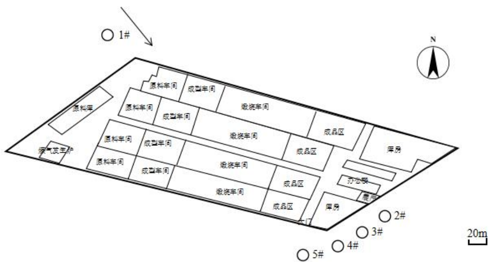
图3-4 隧道窑废气总排放口监测点位示意图
