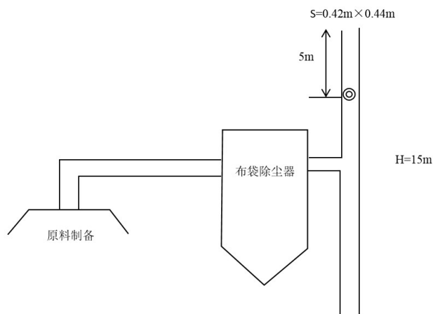
图3-1 1#原料破碎废气排放口监测点位示意图
